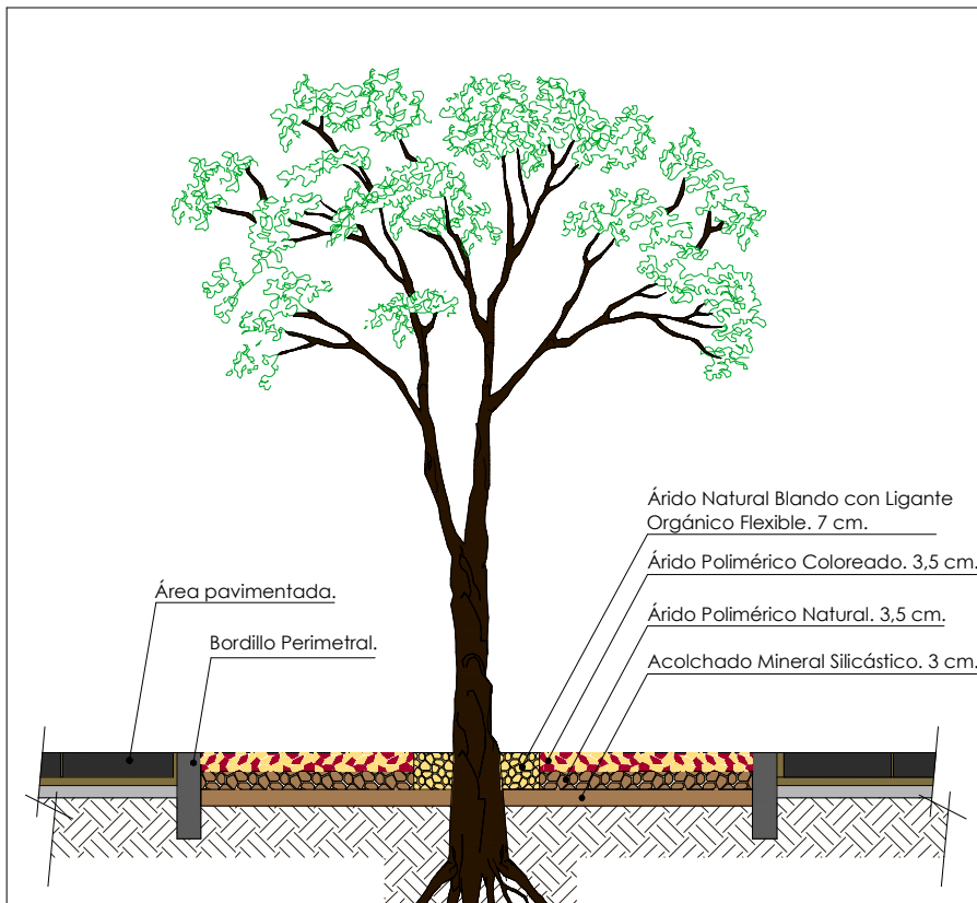
ALCORQUE DRENANTE de 10 cm. de ESPESOR, SISTEMA "Stone Drain®"
